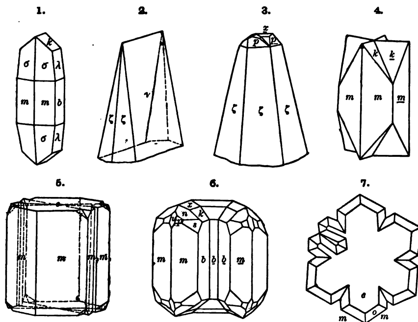
Fig. 1, Kamsdorf, Schmidt-Schrauf. 2, 3, Hüttenberg, Zeph. 4, Molina, Schrauf. 5, Herengrund, Id. 6, Horschenz, Id. 7, Oberstein, Lasp.
