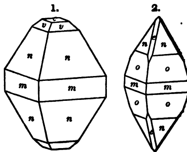
Fig. 1, Des Cloizeaux. Fig. 2, Lévy.
