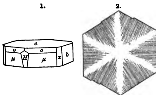
Figs. 1, 2, Zinnwald, Tschermak.
