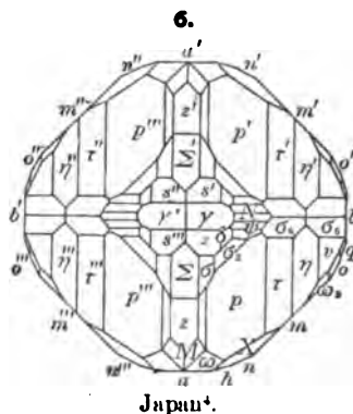
Japan*.
