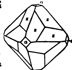
Cuprite.
