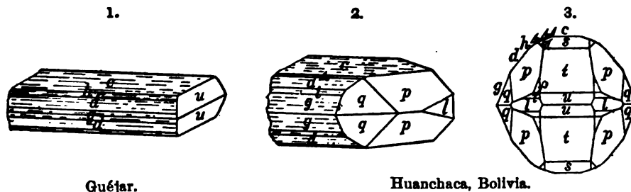
Guéjar.
