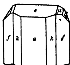
Sjögren .
