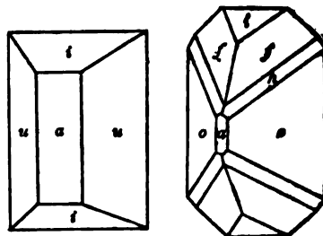
Synadelphite, Sjögren.
