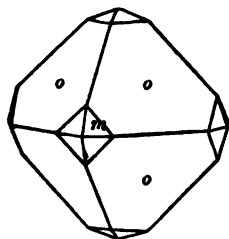
Pajsberg, Flink.
