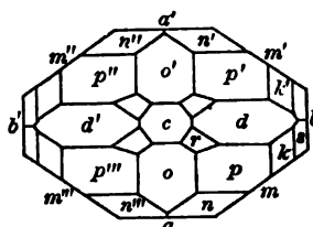
Freiberg, Dbr.
