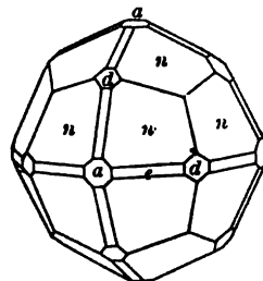
Långban, Flink.
