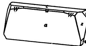
Leadhills, Schrauf.
