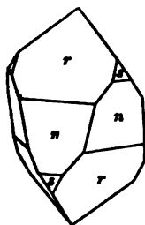
Seligmann.
