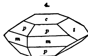
4, Ehrenfriedersdorf.
