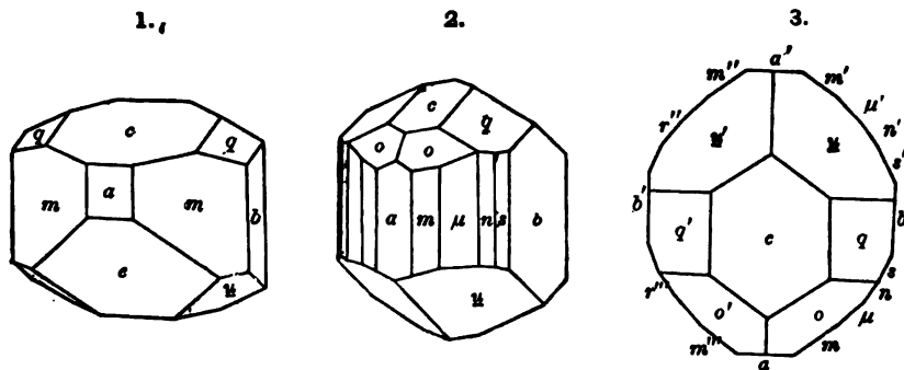
Figs. 1-3, Aschersleben, Luedecke.
