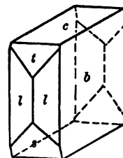
Wyoming, Pirsson.
