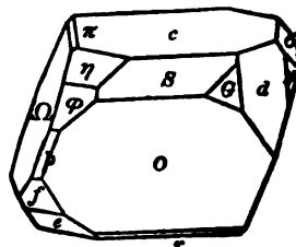
After Schrauf.
