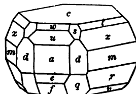
Sardinia, Laspeyres.
