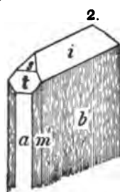
Colorado.
