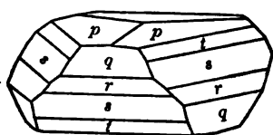
Bereghszasz, Breithaupt.
