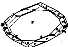
Datolite.
