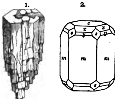
Nerchinsk, Erem.
