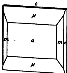
Aranyer Berg.
