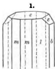
Norwich.
