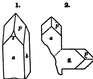
Fig. 1, 2, Cesàro.
