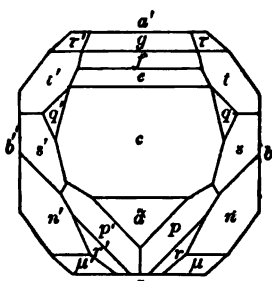
After Scacchi.
