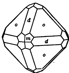
Miask, Kk.
