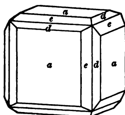
Sarrabus, Klein.
