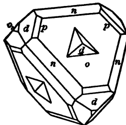
Lölling, Zeph.
