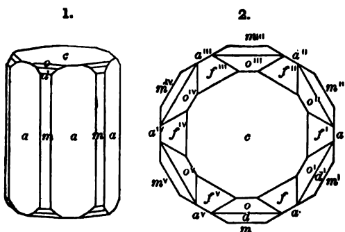
Figs. 1, 2, Långban, Flink.
