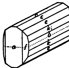
Bertrandite.
