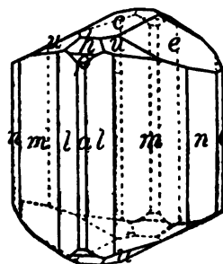
Krennerite.
