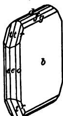
Schrauf.
