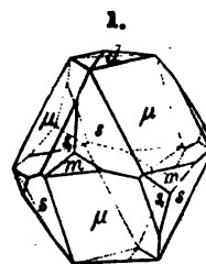
Phenacite.
