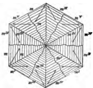
Des Cloizeaux.
