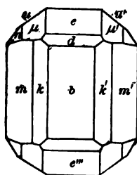
After Scacchi.
