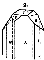
Bodenmais.
