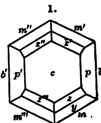
Andreasberg?, Mr.
