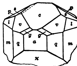
Lorandite, Gdt.
